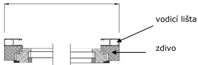
Celková šířka rolety
